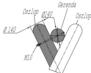
7. ábra Oszlop és gerenda rögzítése
